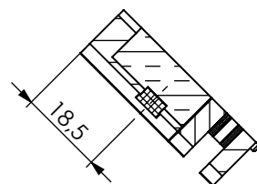
SEZIONE A-A SCALA 1 : 1.5
