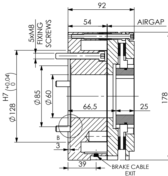
SEZIONE A-A SCALA 1:3
