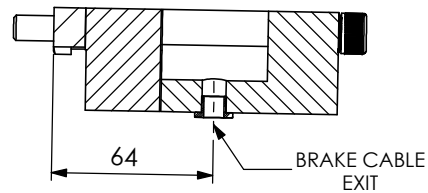
SEZIONE B-B
