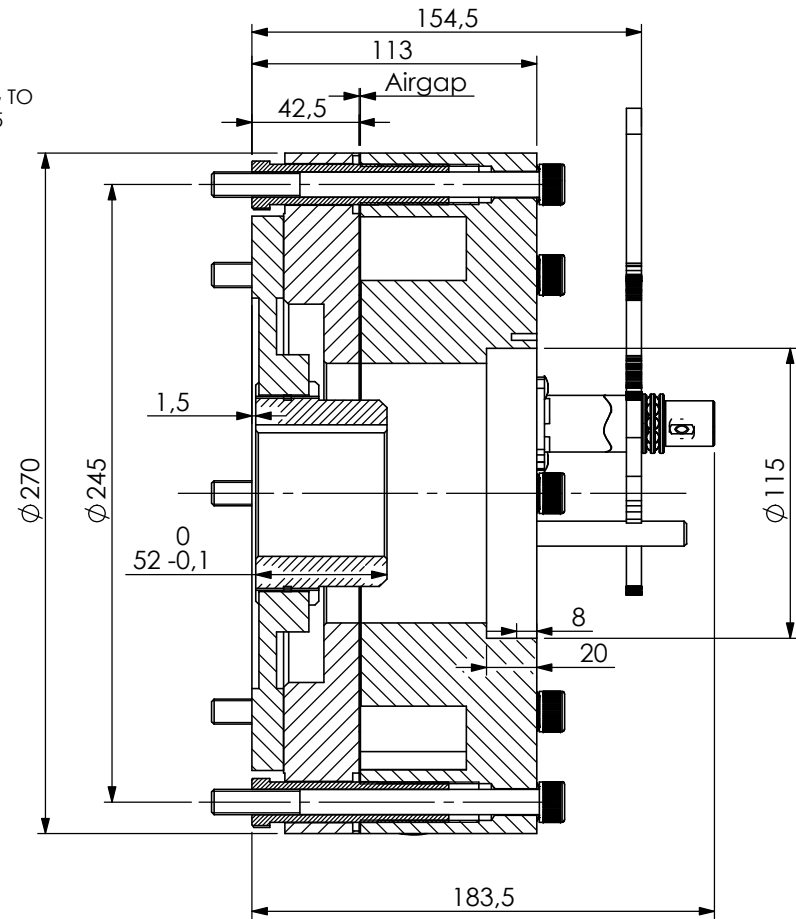
SEZIONE A-A
