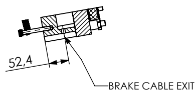
SEZIONE B-B
