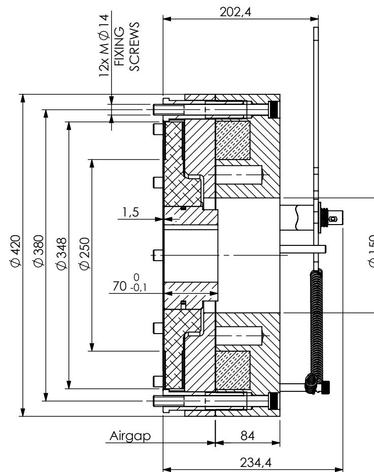
SEZIONE A-A SCALA 1 : 5
