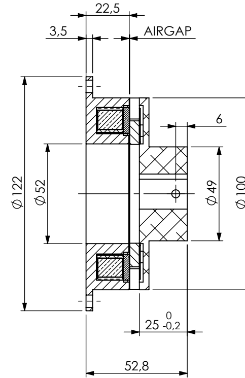
SECTION A-A
