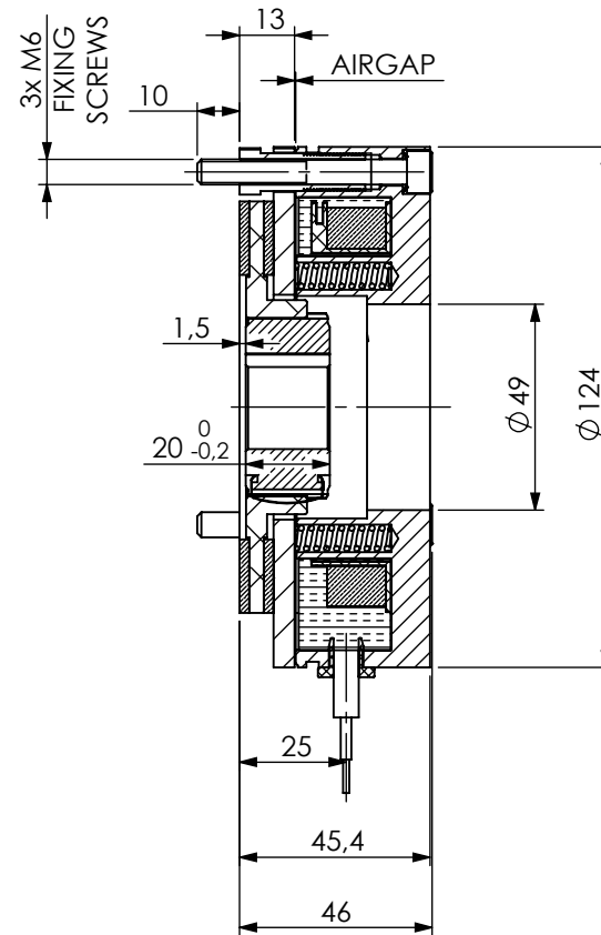
SECTION A-A
